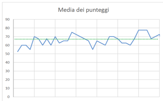
Figura 3 Punteggi SUS per la app "GENnAri" ottenuti durante la sperimentazione, in blu l'andamento dei punteggi ottenuti, in verde è segnalato il valore di soglia (68 punti) oltre il quale si ottengono punteggi superiori alla media
